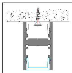
MONTAGGIO A SOFFITTO CEILING-MOUNTING
