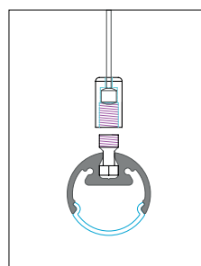
KIT SOSPENSIONE CON SET COPRICAPO SUSPENSION KIT WITH COVER SET
